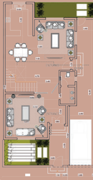
GROUND FLOOR الطابق الأرضي
